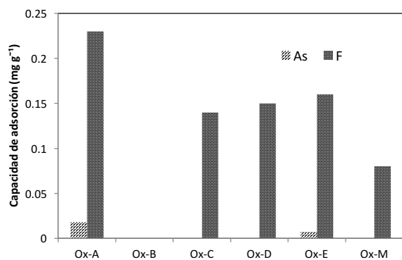
Fig. 2. Capacidad de adsorción de arsénico y fluoruro sobre los óxidos de hierro naturales, concentración inicial de 200 \mu\text{g L}^{-1} y 2.5 \text{ mg L}^{-1} , respectivamente a pH 7 y 25^\circ\text{C} .
