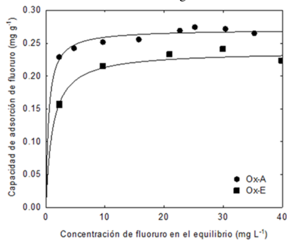
Fig. 4. Isotherma de adsorción de fluoruros en solución acuosa sobre Ox-A y Ox-E a pH 7 y 25^\circ\text{C} , las líneas sólidas indican el modelo de Langmuir.
