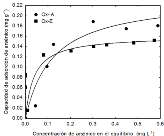
Fig. 3. Isotherma de adsorción de arsénico en solución acuosa sobre Ox-A y Ox-E a pH 7 y 25^\circ\text{C} , las líneas sólidas indican el modelo de Langmuir.
