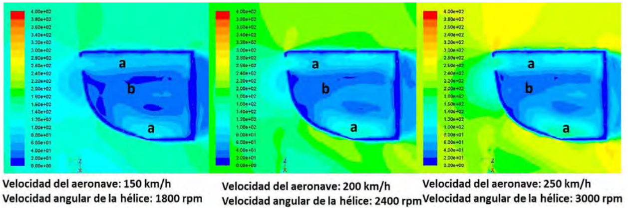
Figura 4.12: Contornos de velocidad en un corte lateral de la cabina de fuego z = 0,14 \text{ m}
