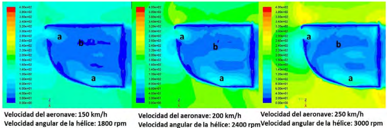
Figura 4.13: Contornos de velocidad en un corte lateral de la cabina de fuego en z = -0,17 \text{ m}
