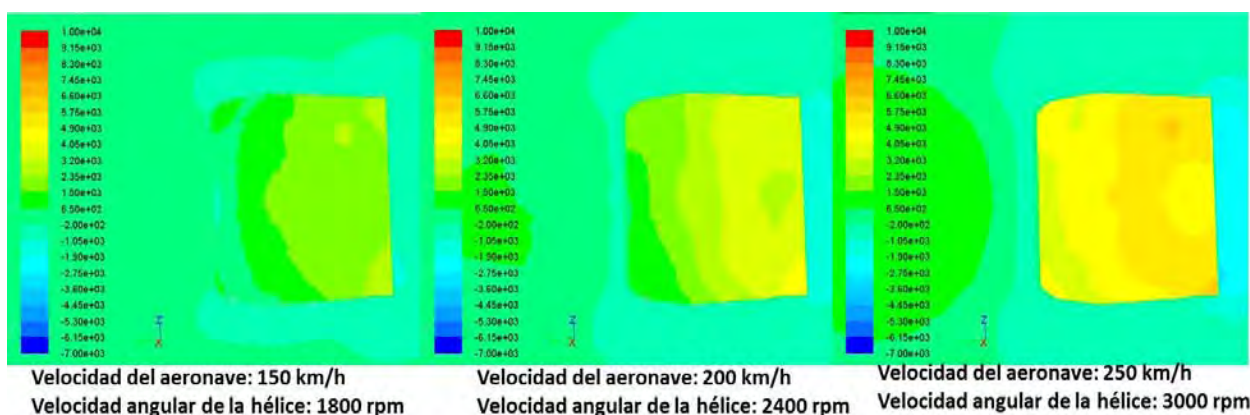
Figura 4.24: Contornos de presión en un corte transversal de la cabina fuego en x = -0,28\text{ m}
