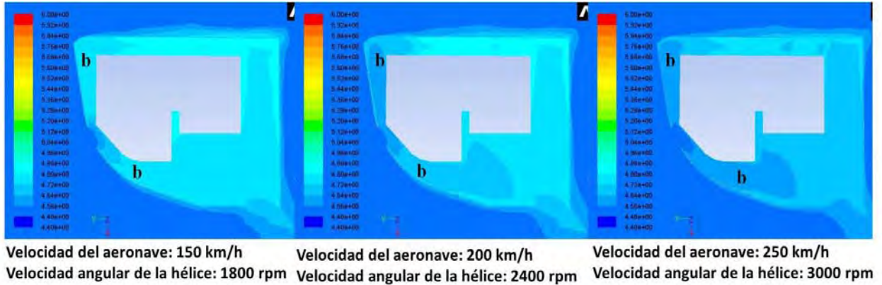
Figura 4.34: Contornos de temperatura en un corte lateral de la cabina de fuego
