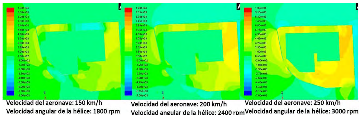
Figura 4.23: Contornos de presión en un corte lateral de la cabina fuego ( z = 0\text{ m} )
