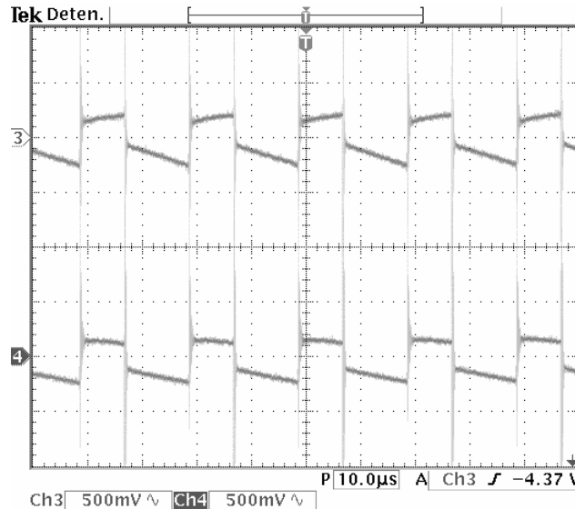
Figura 5.2 Rizos de voltaje de los capacitores del convertidor cuadrático elevador prototipo. (Superior a inferior) Rizo segundo capacitor y rizo primer capacitor (500 mV/div) (Tiempo 10 ms).
