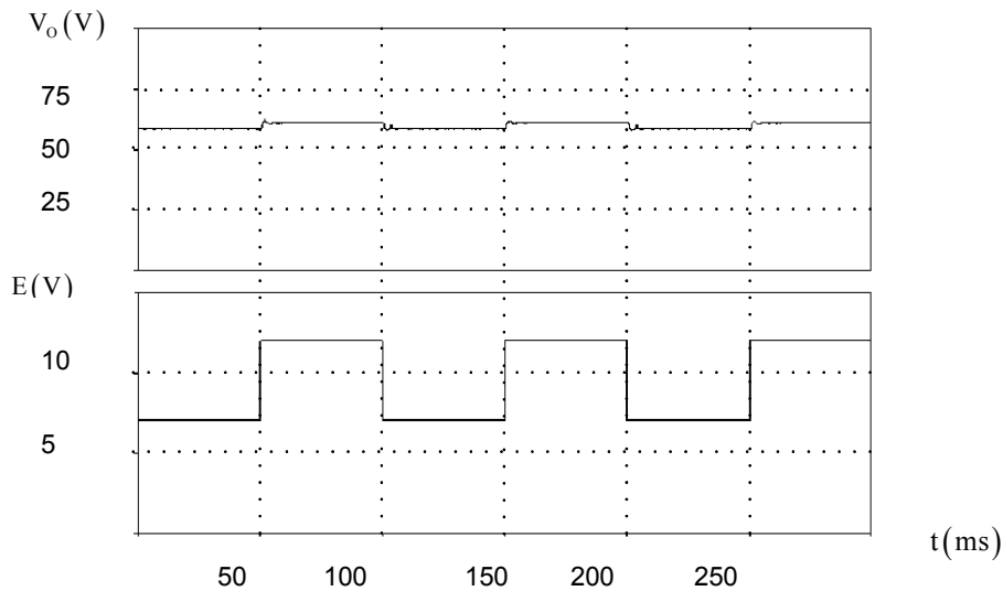
Figura 4.9. Voltaje de salida V_o en lazo cerrado para cambios en el voltaje de entrada de 7 V a 12 V. ( Superior a inferior ) Voltaje de salida y voltaje de entrada: (25 V/div, 5 V/div), (Tiempo: 50 ms).
