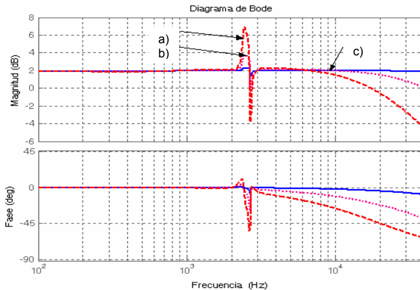
Figura 4.14 Respuesta en frecuencia de la función de transferencia \tilde{I}_{L_1}(s)/\tilde{v}_{control}(s) para diferentes valores de K_p : a) 3.67 \times 10^3 , b) 8.8 \times 10^3 , y c) 4.4 \times 10^4
