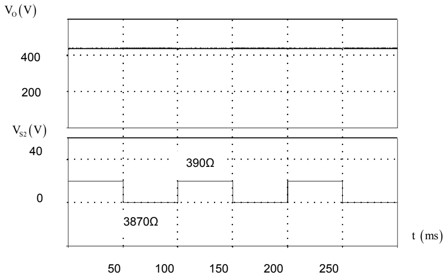
Figura 4.20. Respuesta transitoria para cambios tipo escalón en la carga entre 390 \Omega y 3870 \Omega en lazo cerrado. (Superior a inferior) Voltaje de salida y señal de voltaje a la compuerta del interruptor MOSFET para cambio de carga. (200 V/div, 40 V/div), (Tiempo: 50 ms).
