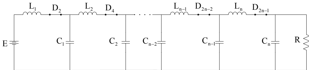
Figura 2.6. Circuito del convertidor elevador de n-etapas con el interruptor activo abierto.
