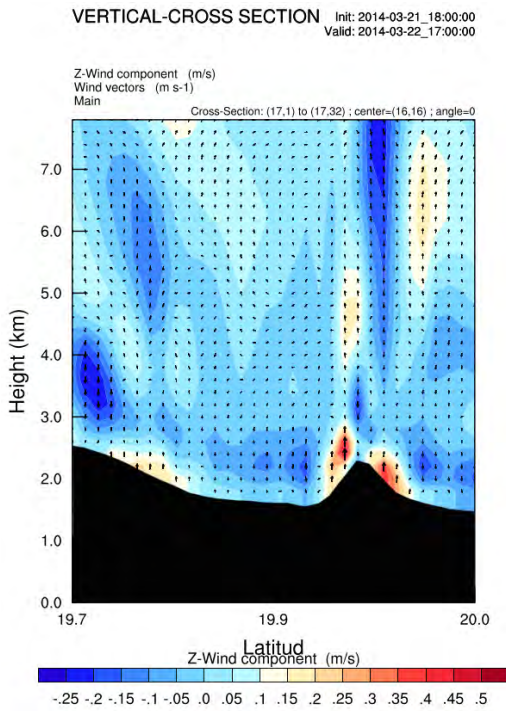
Figura 3.51 Corte vertical de terreno con distribución de vorticidad potencial con vapor de agua en porción de mezcla (a y b) y velocidad del viento en Z con vectores de viento (c y d) en D3.
