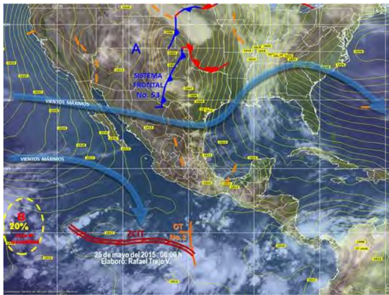
Figura 1.4 Imagen interpretada del satélite GOES para las 06:00 horas.
