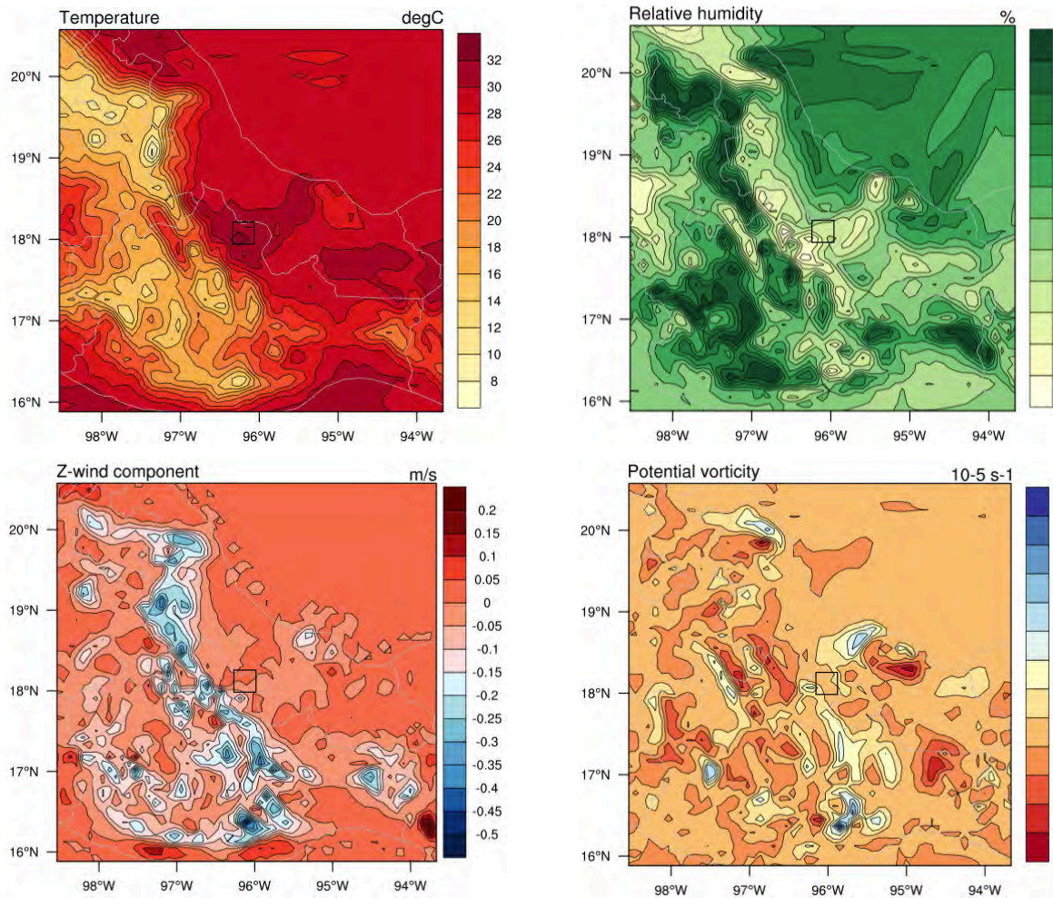
Figura 3.55 Distribución de temperatura (a), humedad relativa (b), velocidad del viento en Z (c) y vorticidad potencial (d) a nivel del suelo.
