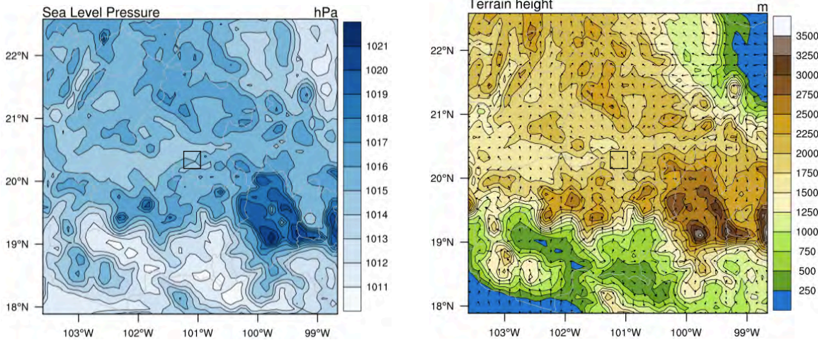
Figura 3.35 Distribución de presión a nivel del mar (a) y topografía con vectores de viento (b) a nivel del suelo.
