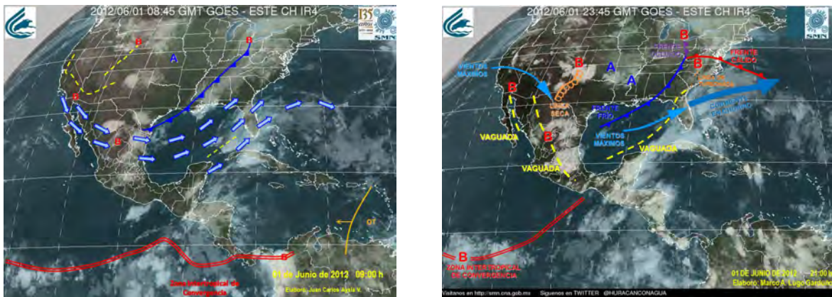
Figura 3.12 Imágenes interpretadas del Satélite GOES para las 09:00 y 21:00 horas.
