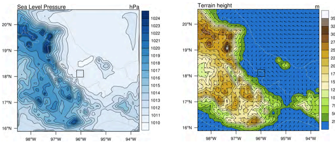
Figura 3.56 Distribución de presión a nivel del mar (a) y topografía con vectores de viento (b) a nivel del suelo.
