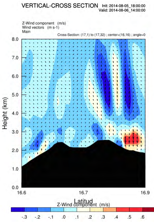
Figura 3.65 Corte vertical de terreno con distribución de vorticidad potencial con vapor de agua en porción de mezcla (a y b) y velocidad del viento en Z con vectores de viento (c y d) en D3.
