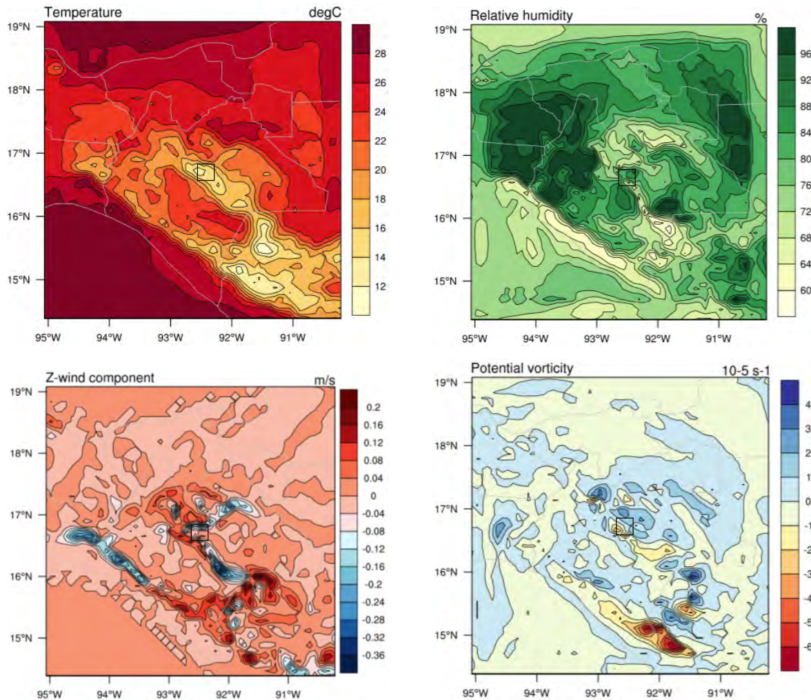
Figura 3.62 Distribución de temperatura (a), humedad relativa (b), velocidad del viento en Z (c) y vorticidad potencial (d) a nivel del suelo.
