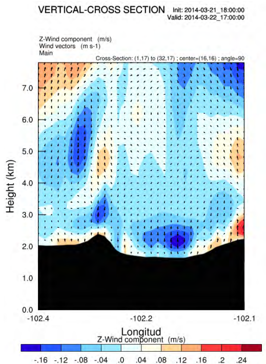
Figura 3.51 Corte vertical de terreno con distribución de vorticidad potencial con vapor de agua en porción de mezcla (a y b) y velocidad del viento en Z con vectores de viento (c y d) en D3.
