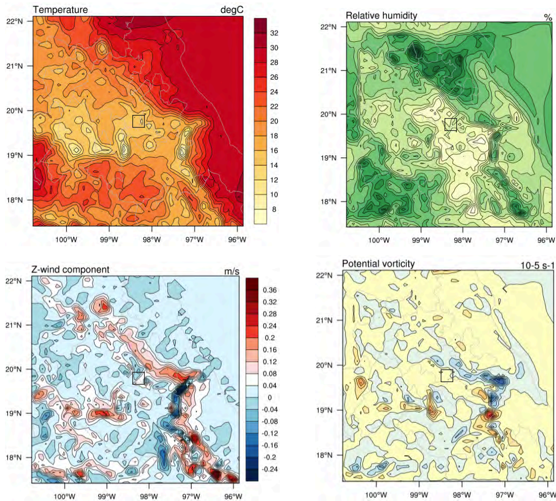
Figura 3.69 Distribución de temperatura (a), humedad relativa (b), velocidad del viento en Z (c) y vorticidad potencial (d) a nivel del suelo.
