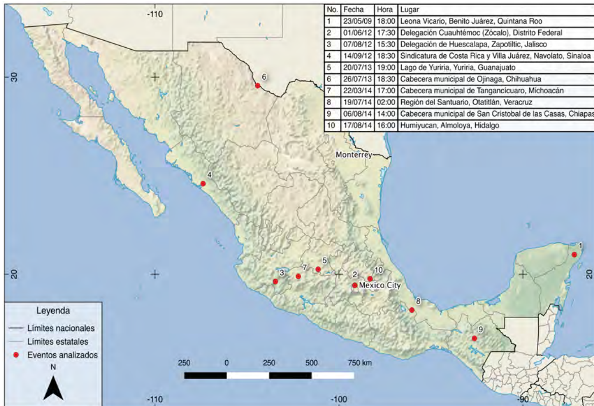
Figura 3.2 Distribución espacial de los casos analizados. Elaboración propia.
