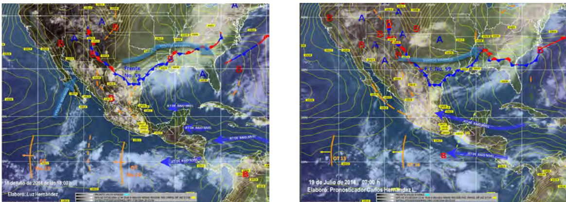
Figura 3.54 Imágenes interpretadas del Satélite GOES para las 07:00 y 19:00 horas.
