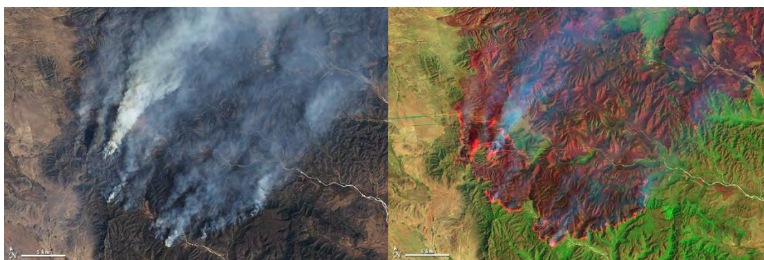
Figura 1.7 Incendios El Bonito y La Sabina al norte de México en el estado de Coahuila. a) muestra densas plumas de humo hacia el noreste, b) incluye infrarojo y luz visible, muestra una vista a través del humo el terreno recientemente quemado. Imagen tomada por el satélite
